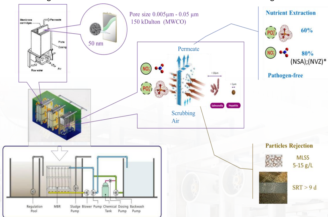
Figure 1: Schéma de fonctionnement du système
